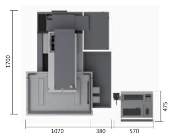
平面
