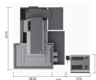
平面
